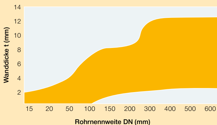
Abmessungsspektrum für die Fertigung von Rohren aus Band
